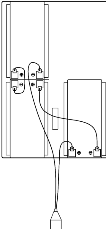
Рисунок 7 — схема соединений АКБ
